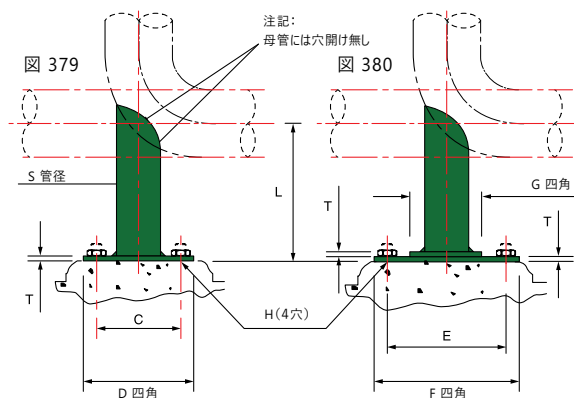
固定ベースサポート / スライディングベースサポート – 図 379H、379E、380H、380E
