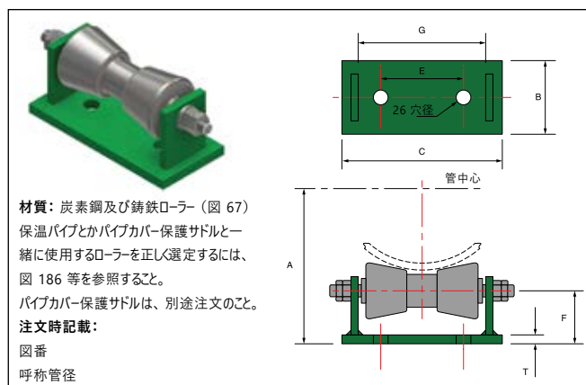
パイプローラー及びスタンド - 図 39
