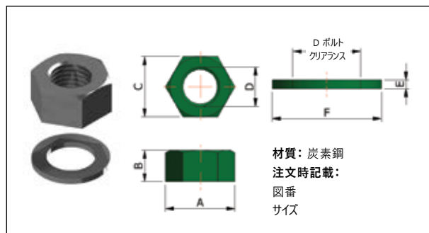
図 165 - 六角ナット
