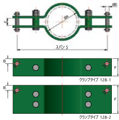
ライザークランプ – 図 128
