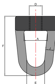
無溶接アイハット・右・左ネジ – 図 279L、279R
