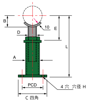
調整型パイプサポート – 図 101
