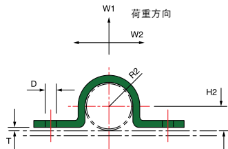
図319Aアンカー
