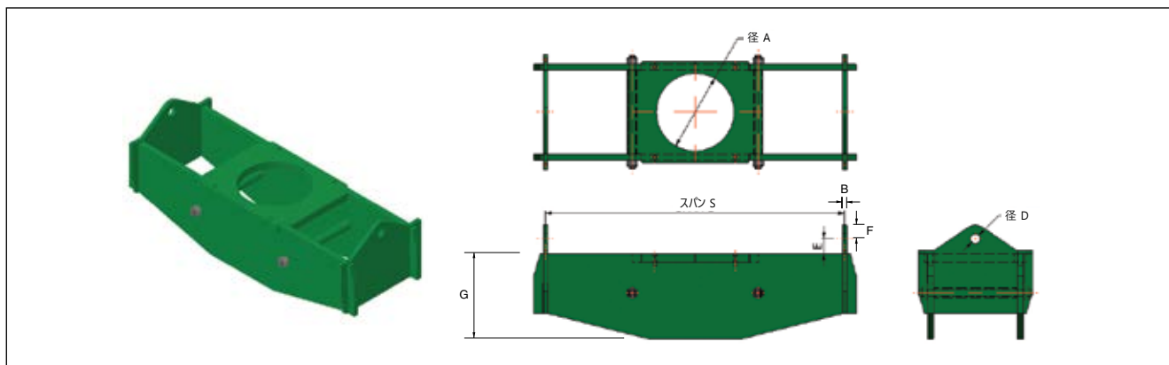
平板型ライザーランプ – 図 129
