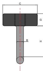
無溶接アイハット・右・左ネジ – 図 279L、279R
