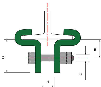
ビームクランプ – 図 15
