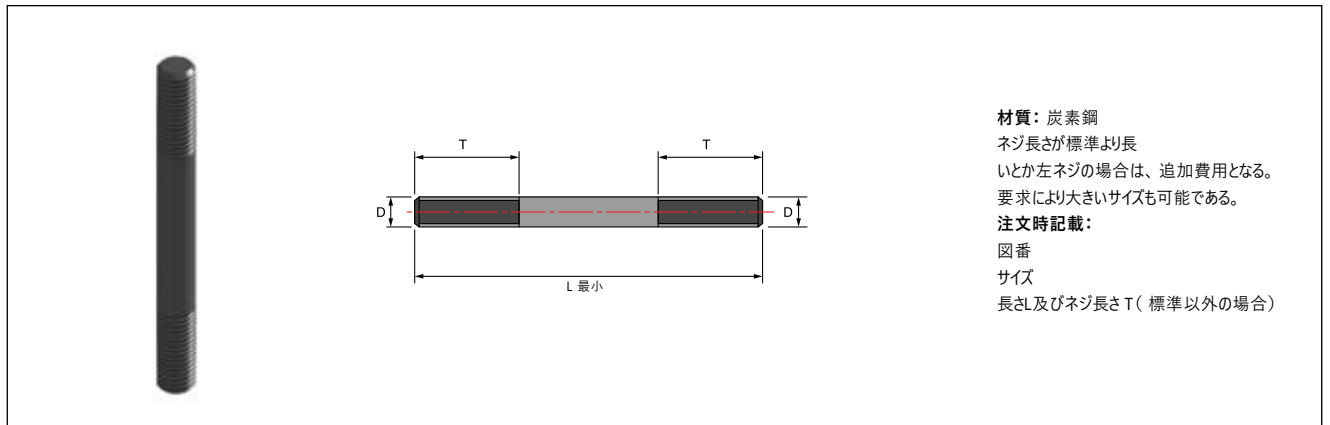
両端ネジロッド – 図 133
