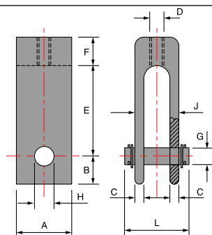
クビス (鋼製) – 図 276P
