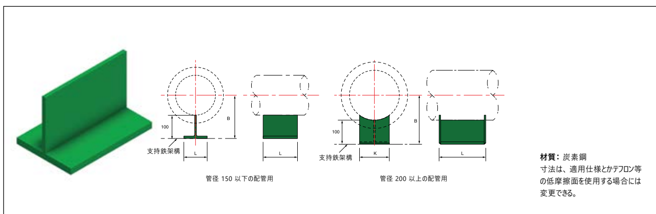
溶接型スライディングシュー (ガイド付き) – 図 382
