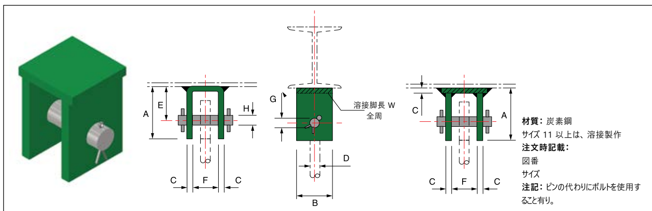
ビームウェルディングアタッチメント－図 113B
