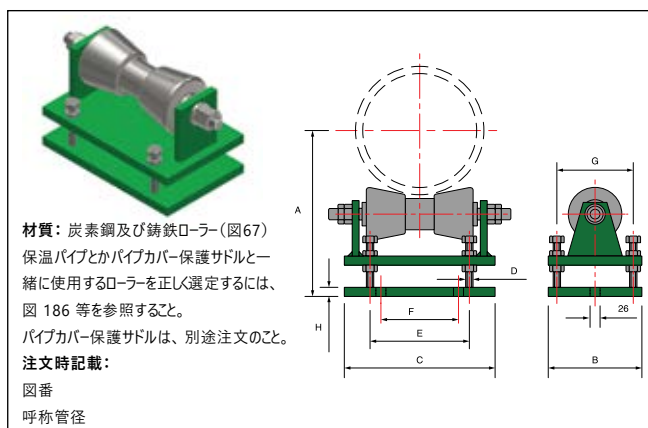
パイプローラー及び調整型スタンド - 図 40
