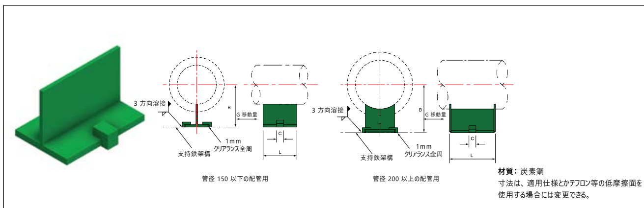
溶接型スライディングシュー (ガイド付き) – 図 382
