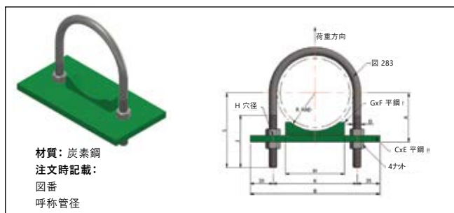
アンカーチェアー - 図 127 (100-600)
