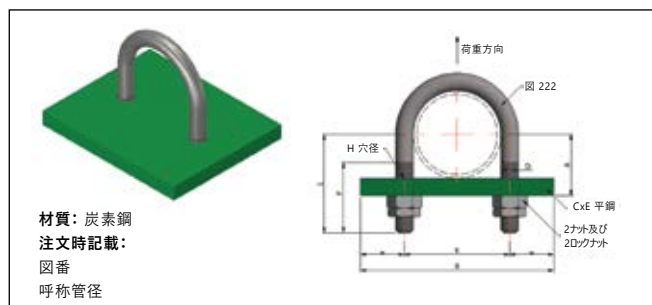
アンカーチェアー - 図 127 (20-90)
