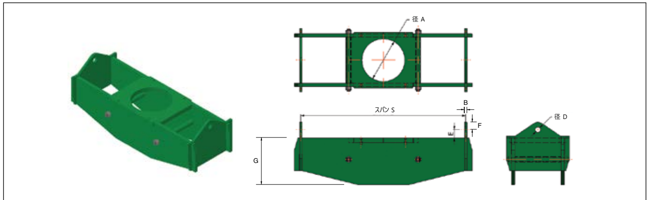
平板型ライザークランプ – 図 129
