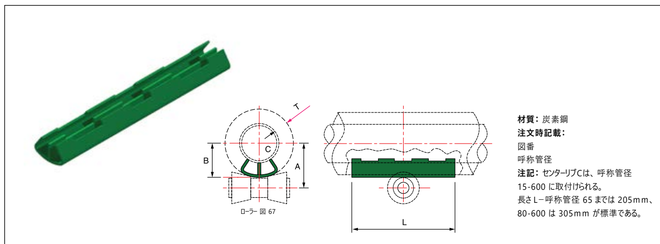
パイプカバー保護サドル – 図 186
