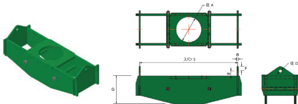
平板型ライザーランプ – 図 129
